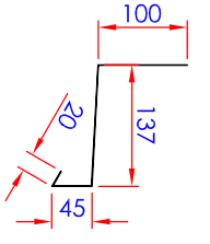
Plastisol Coated Cill Solent Blue (D)
